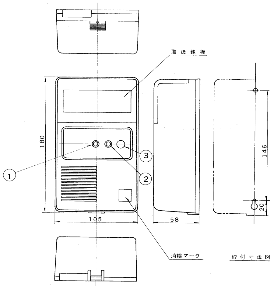
外觀寸法図
