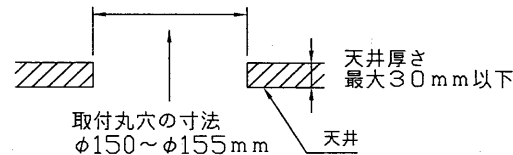
取付寸法図
