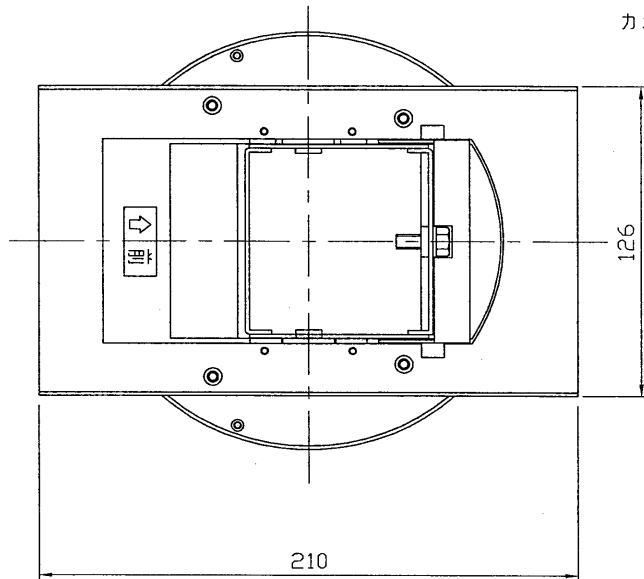
外観寸法図
