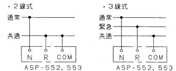
(ASP-552, 553に組み込み時) 結線方法
