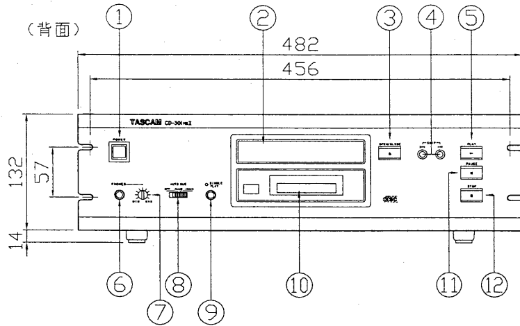
外観寸法図
