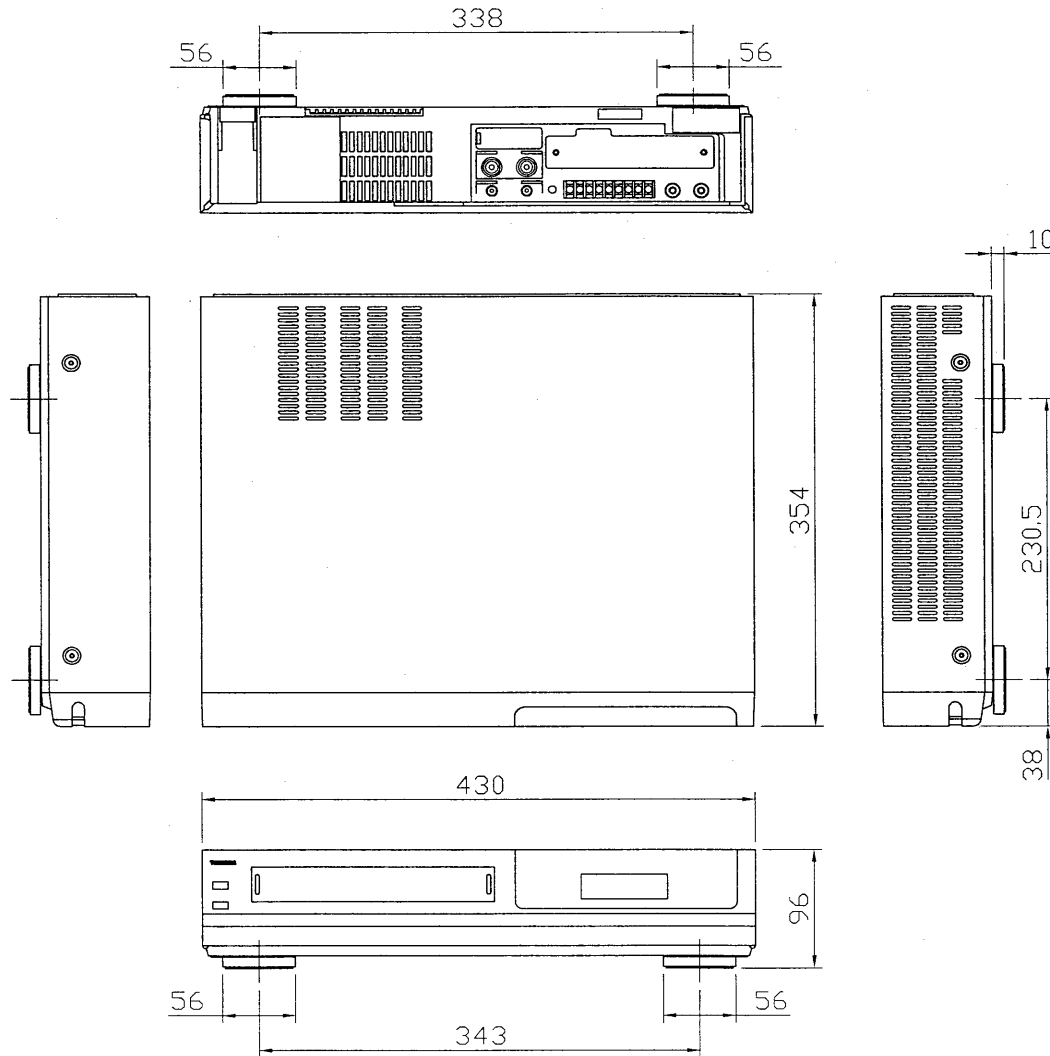
外觀寸法図
