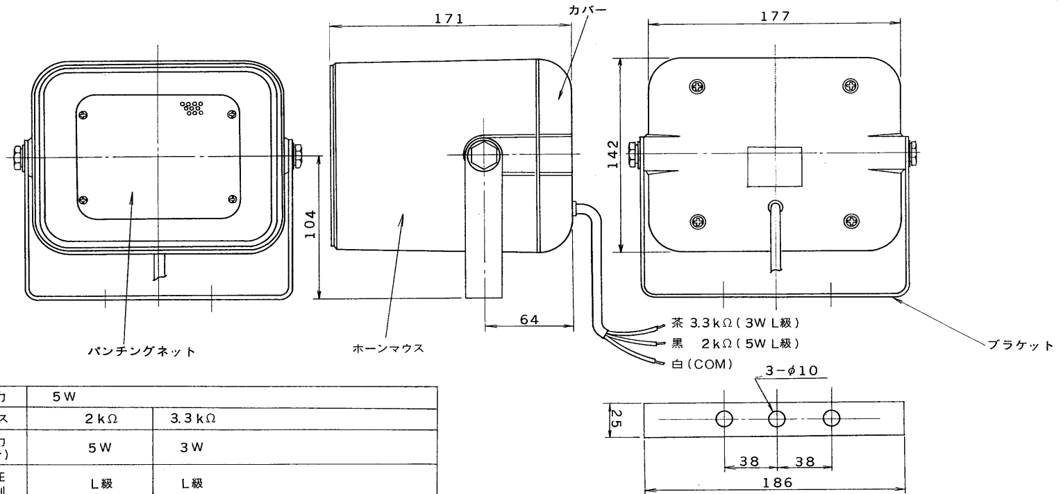
外 観 寸 法 図
