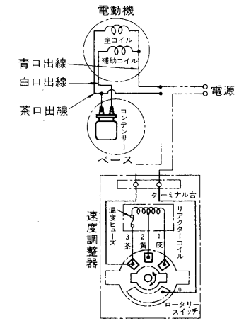
F-691結線図
