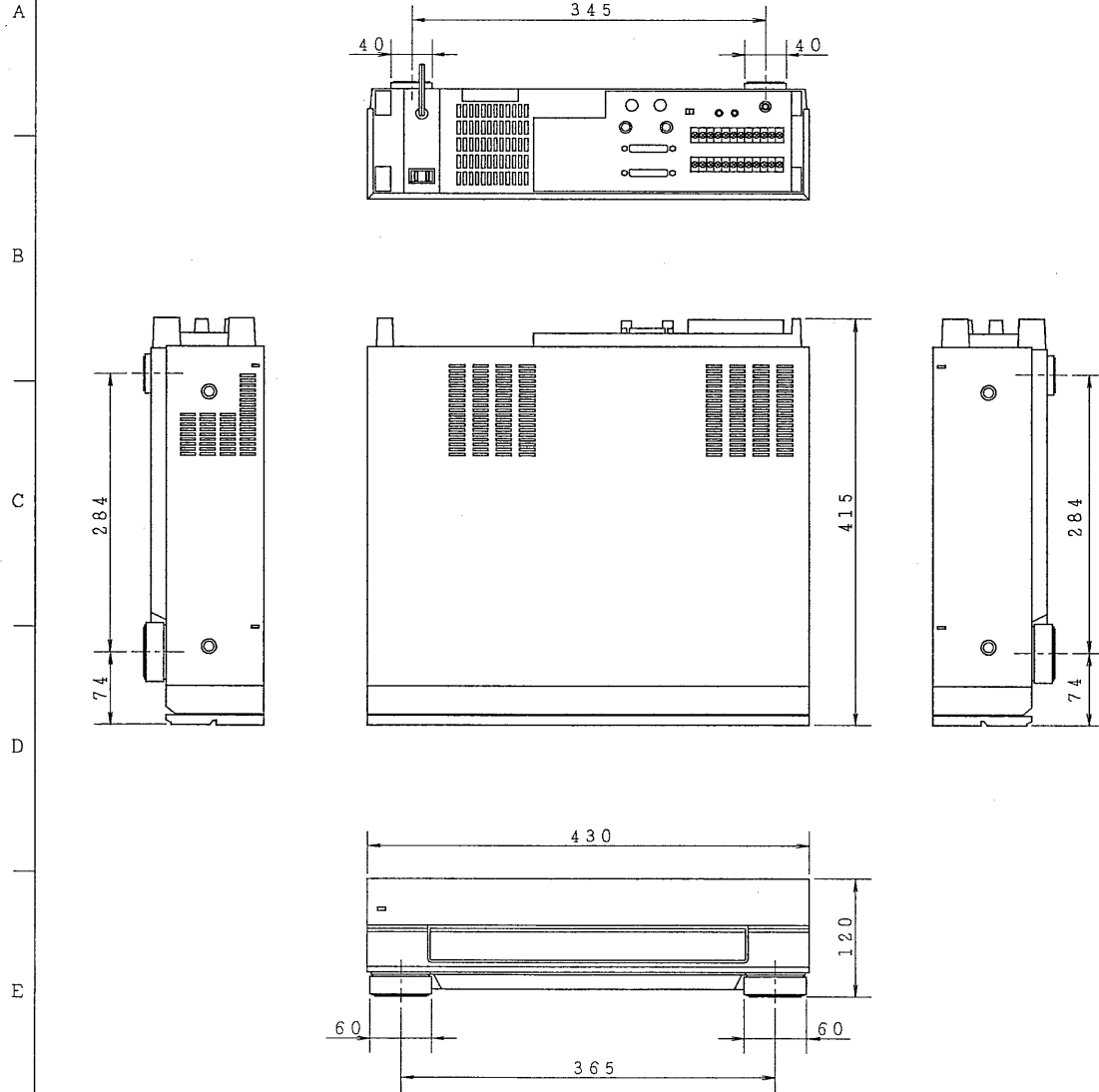
外観寸法図
