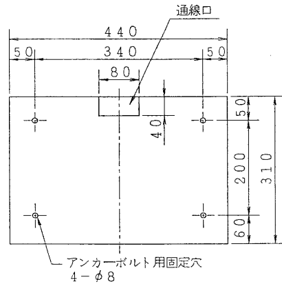
取付寸法図
