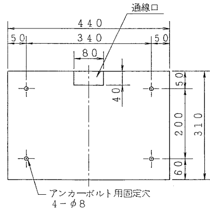
取付寸法図
