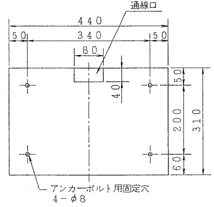
取付寸法図
