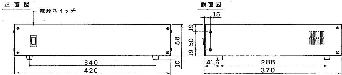
外觀寸法図
