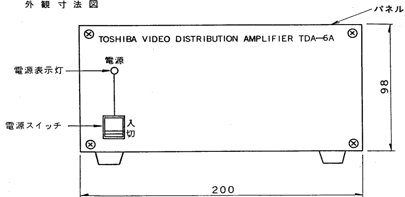
外観寸法図
