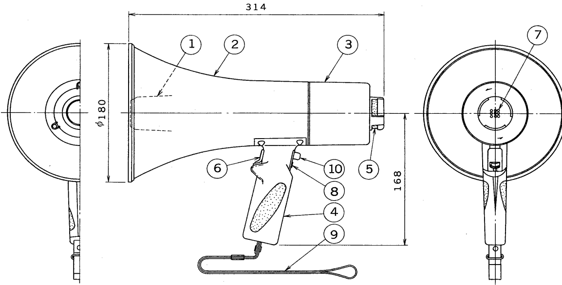
外形寸法図
