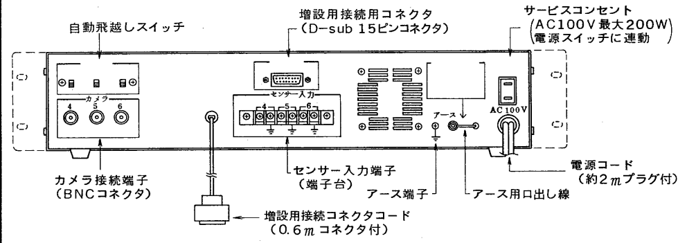
背面図
