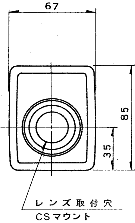
外観寸法図
