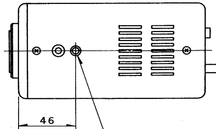
カメラ取付ねじ穴(上下面) 1/4インチ-20UNC×2(深さ10mm)
