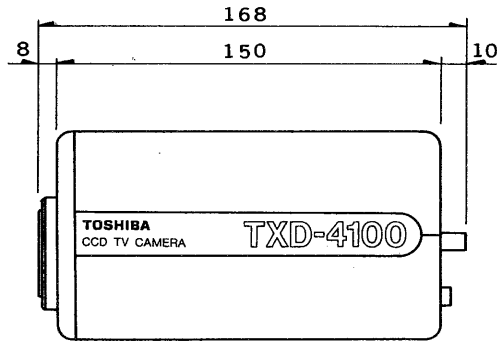
レンズ接続用コネクタ(4P)
