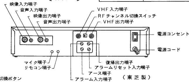
〔背面図〕
