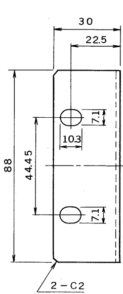
外形寸法図
