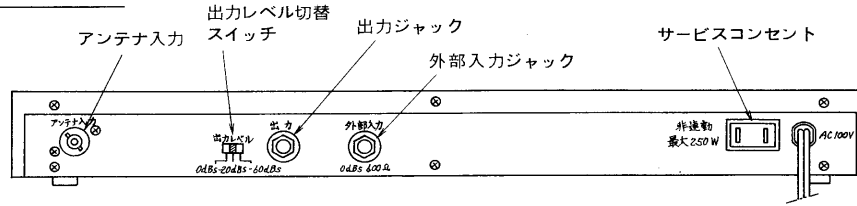
外觀寸法図
