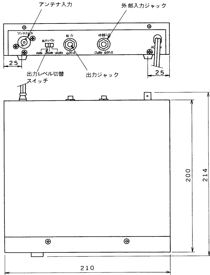
外観寸法図
