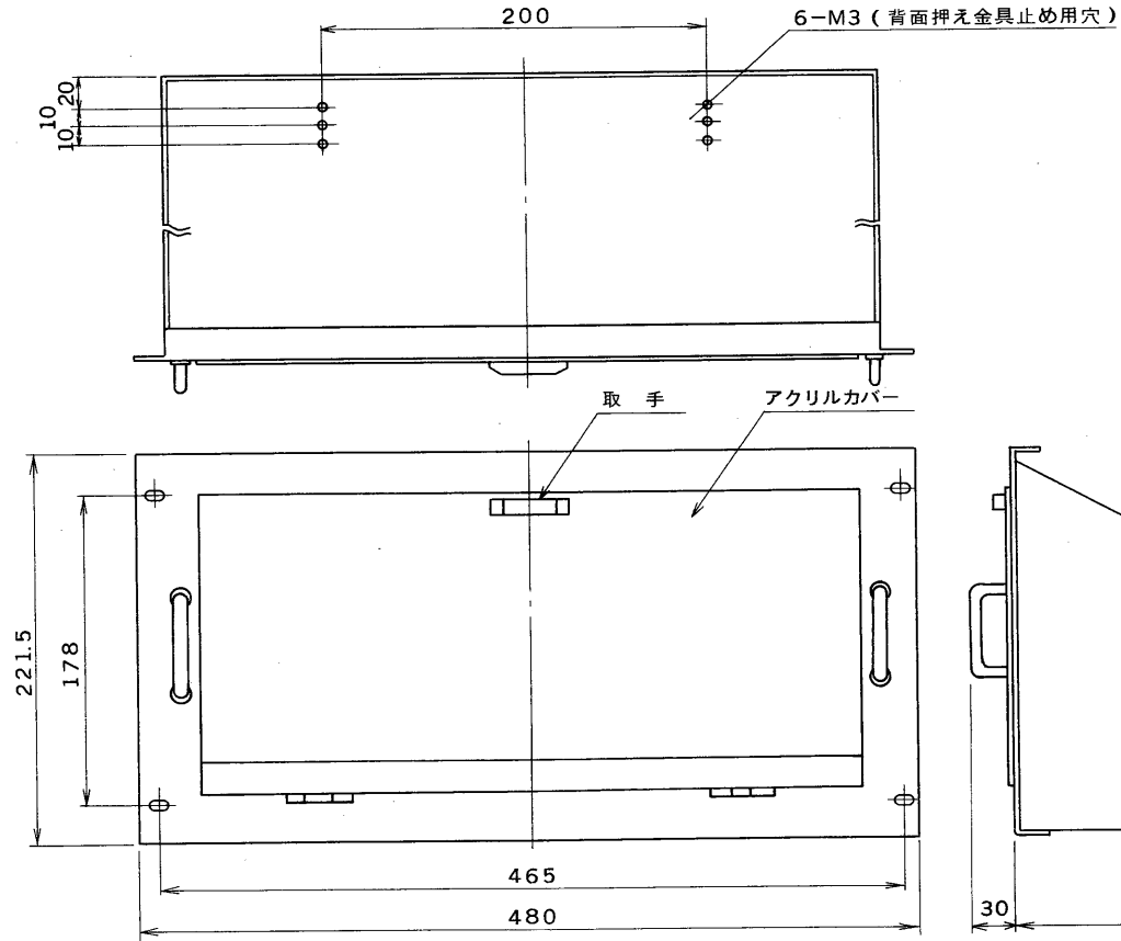
外觀寸法図 (EIA:5U)
