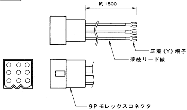
外 観 図
