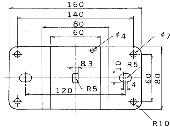
アタッチメント寸法図
