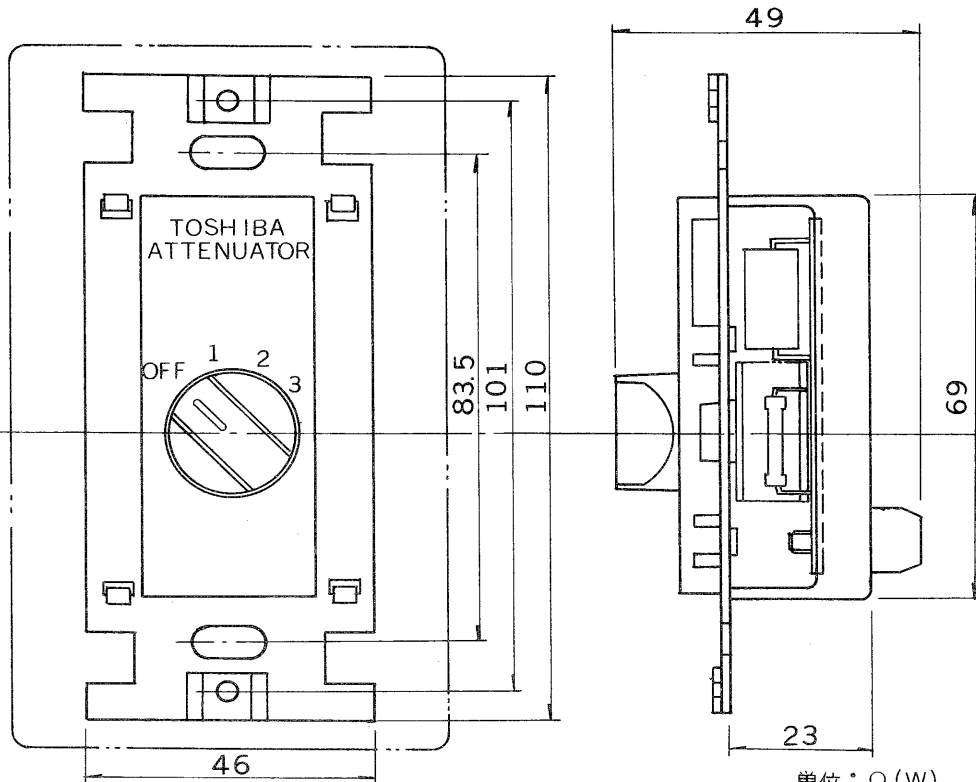
外観寸法図
