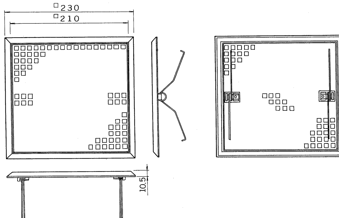
外観寸法図
