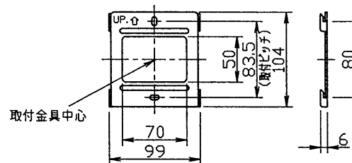
取付金具
