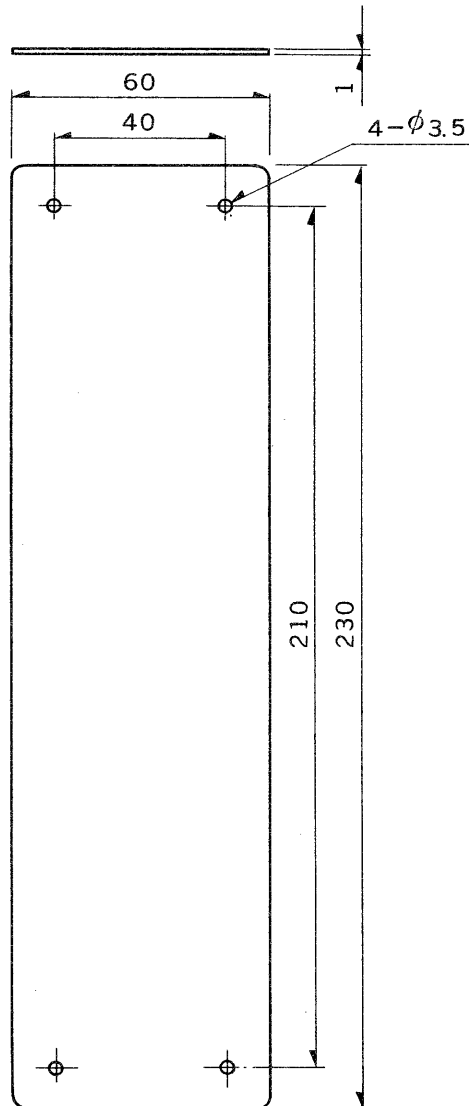
連結金具 (×1)
