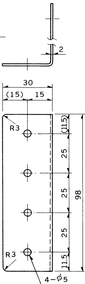
取付金具 (×2)
