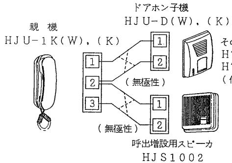
接続例 (最大接続例)
