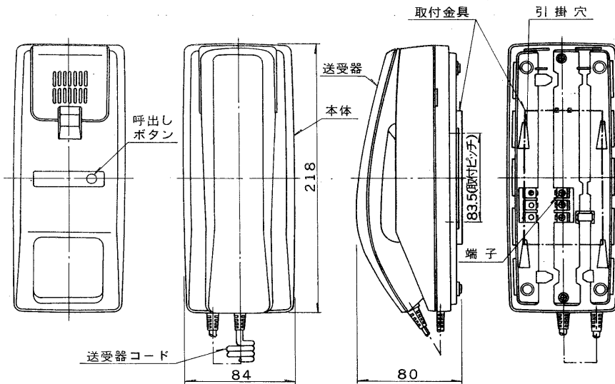
外形図
