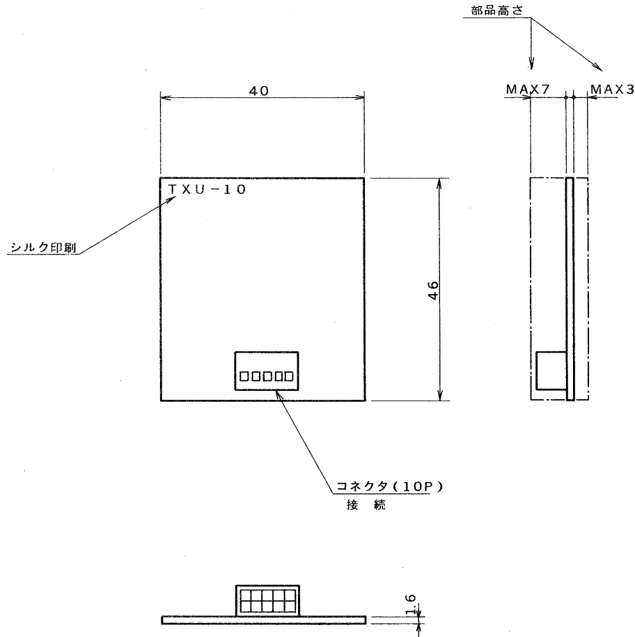
外觀寸法図
