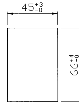
壁の穴あけ寸法
