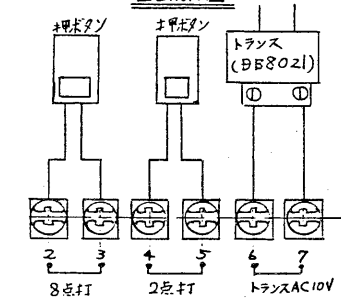
配線図
