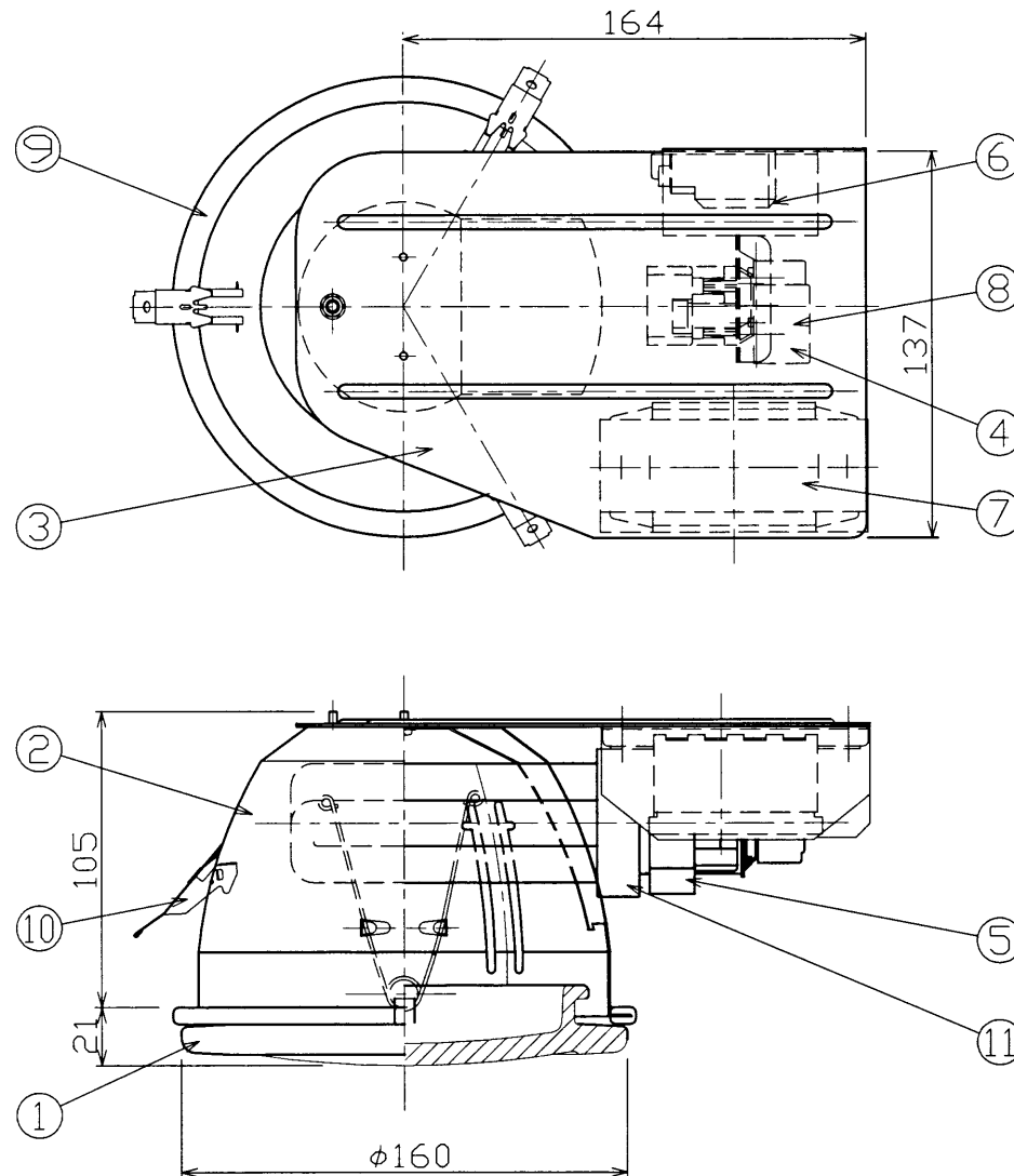
埋込穴寸法 天井取付厚さ：5～25mm
