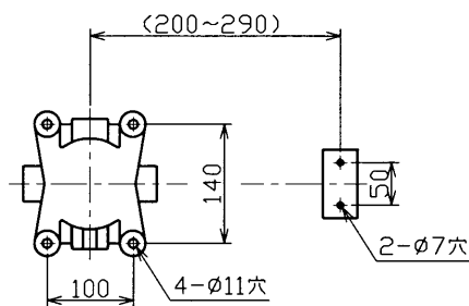
安定器・端子箱取付寸法
