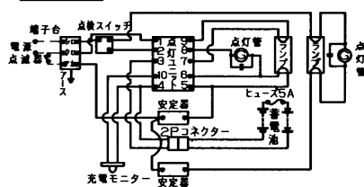
結線図
