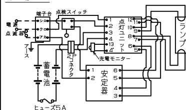
結 線 図
