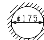
埋込穴寸法 天井取付厚さ: 3~45mm
