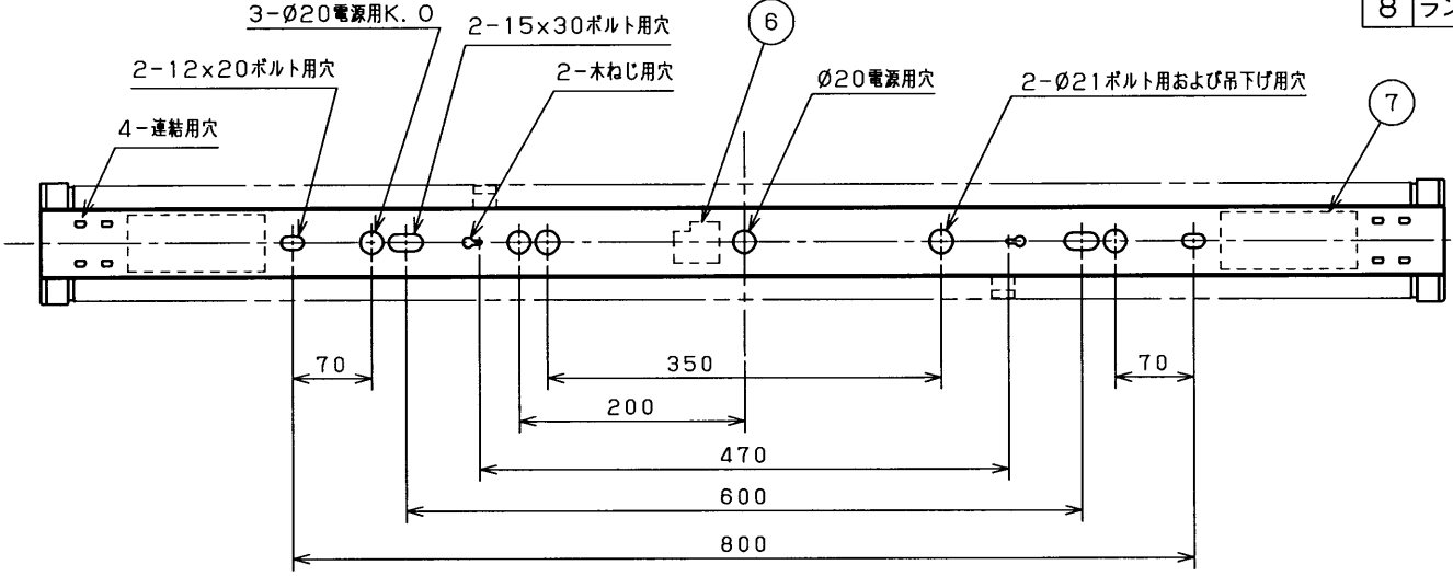
直付連結使用例
