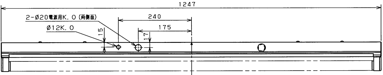
適合連結金具 C-62N (吊下げ専用)
