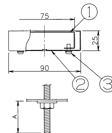
インサートボルト（器具取付ボルト）器具内寸法 注）A寸法は、20mmを超えないようにしてください。
