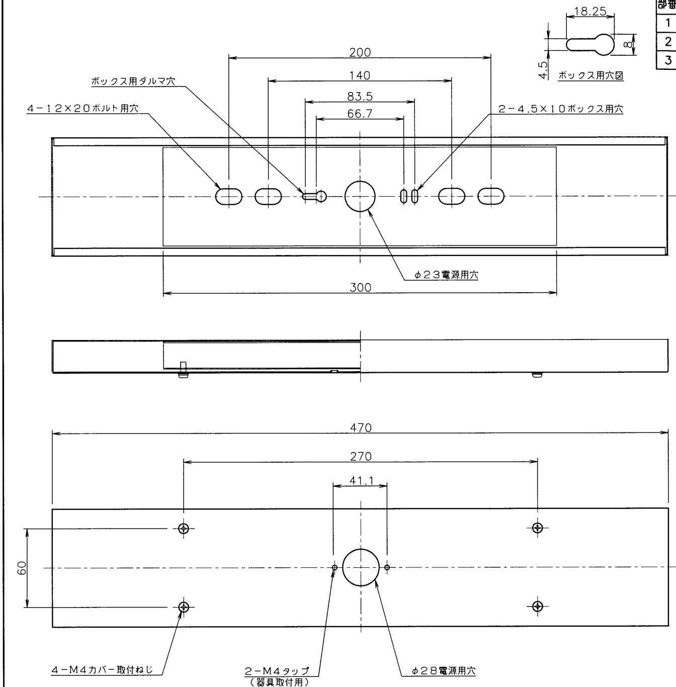
インサートボルト（器具取付ボルト）器具内寸法 注）A寸法は、20mmを超えないようにしてください。
