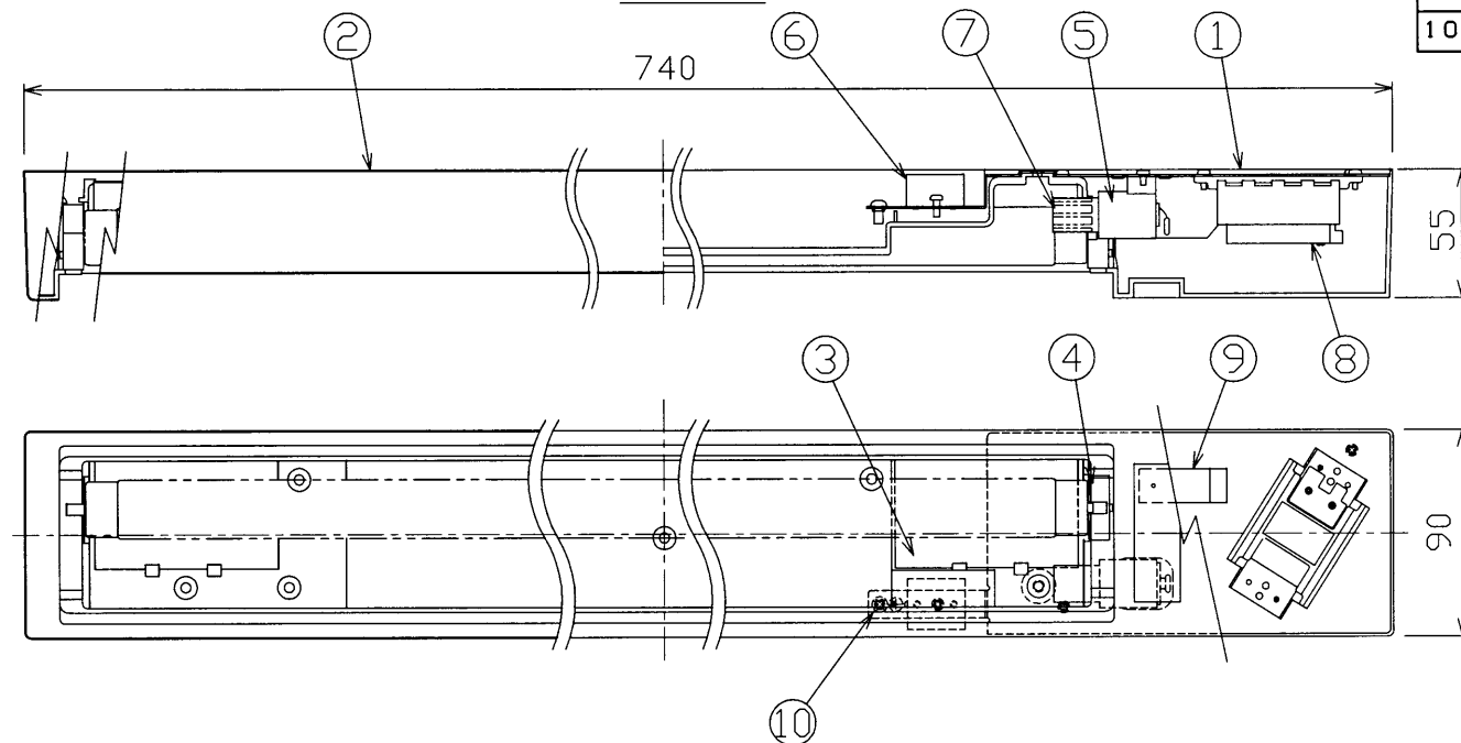
取付寸法図
