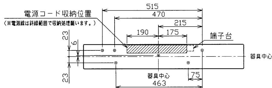
取付寸法図
