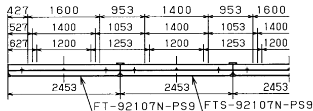
直付連結使用例
