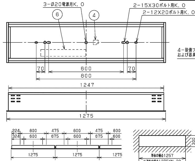
埋込み連結使用例
