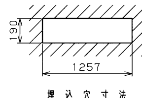
埋 込 穴 寸 法
