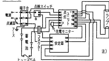
結線図
