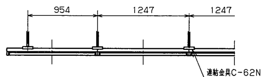
吊下連結使用例
