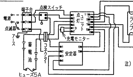
結 線 図
