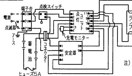
結 線 図
