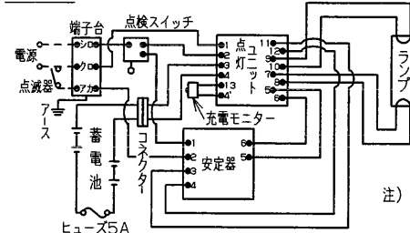
結 線 図
