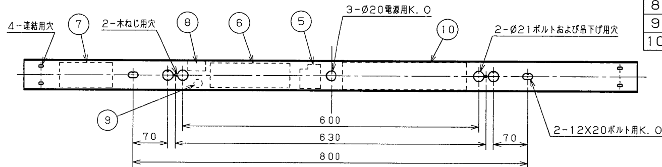
直付連結使用例
