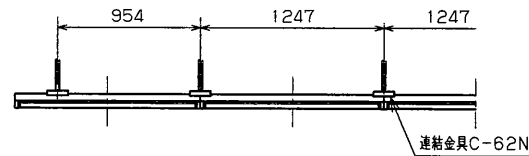
吊下連結使用例
