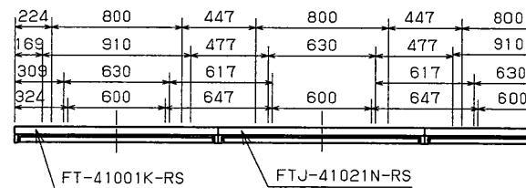
直付連結使用例
