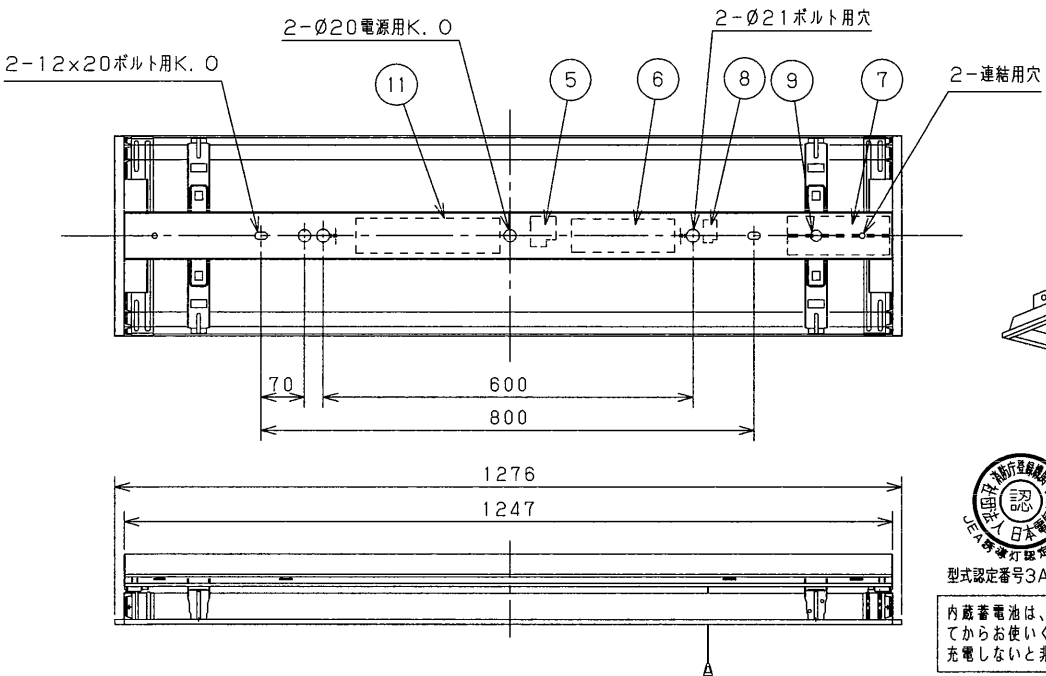
埋込連結使用例
