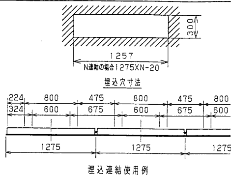
埋込連結使用例
