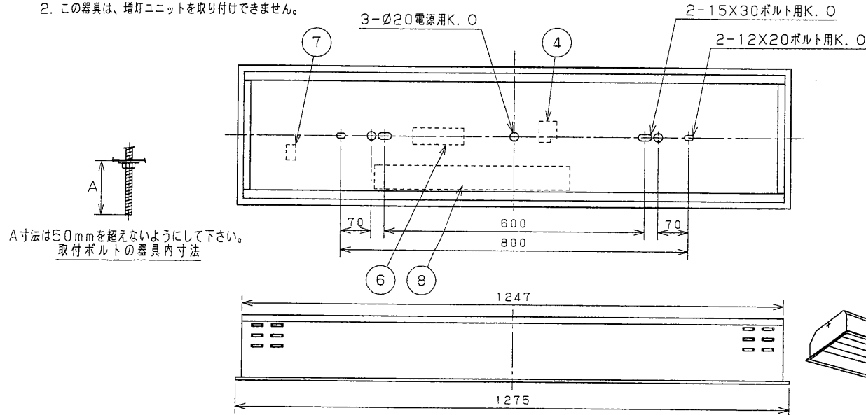
埋込連結使用例
